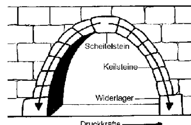
Keilsteinbogenbrücke
